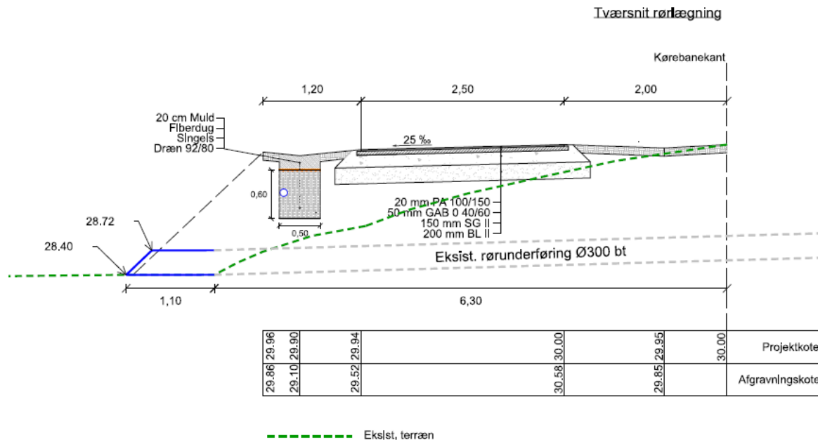
Figur 3: Rørunderføringens placering under den kommende cykelsti
