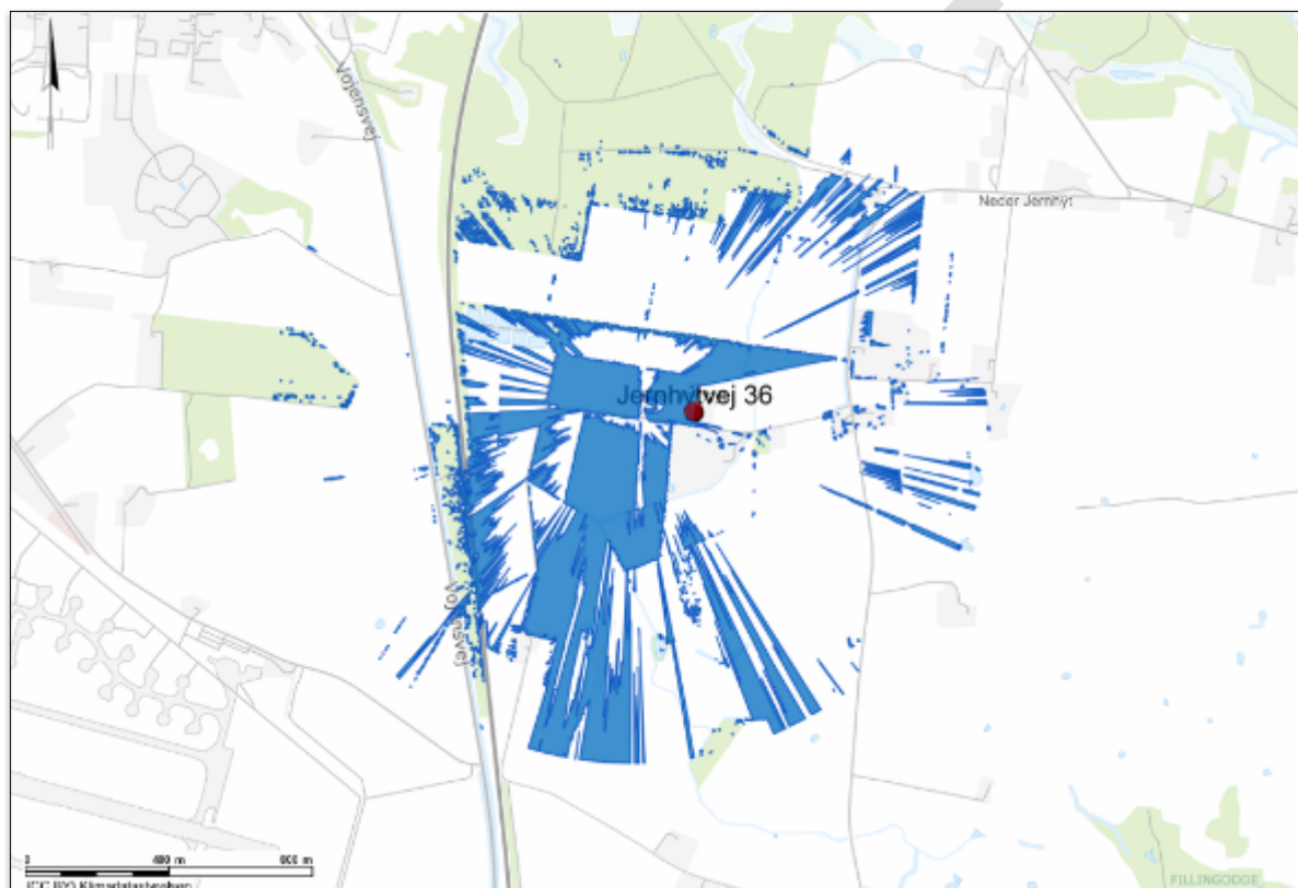
Figur 2 Synlighedsberegning for Ny GB5. Elementhøjde: 13 m. Betragterhøjde: 1,5 m, Radius: 1.000 m
