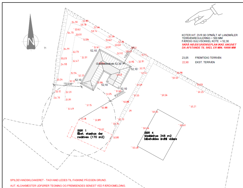
Fra ansøgningen: Situationsplan
