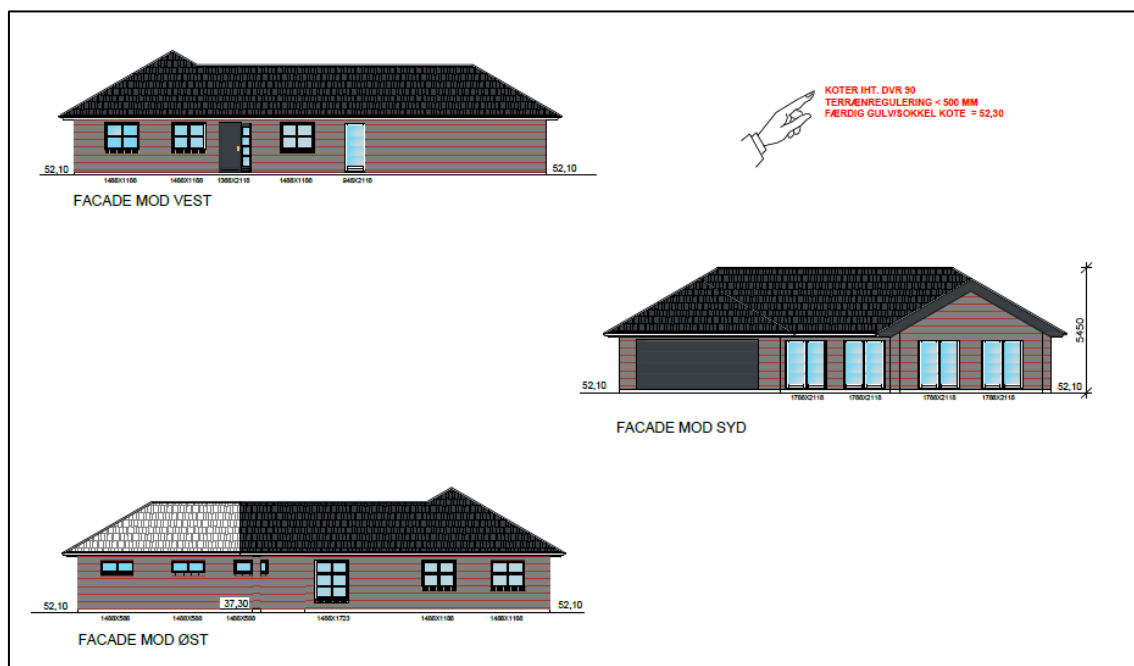
Fra ansøgningen: Facadetegninger mod vest, syd og øst
