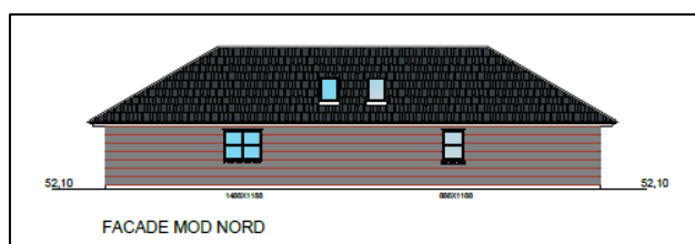
Fra ansøgningen: Facadetegninger mod nord
