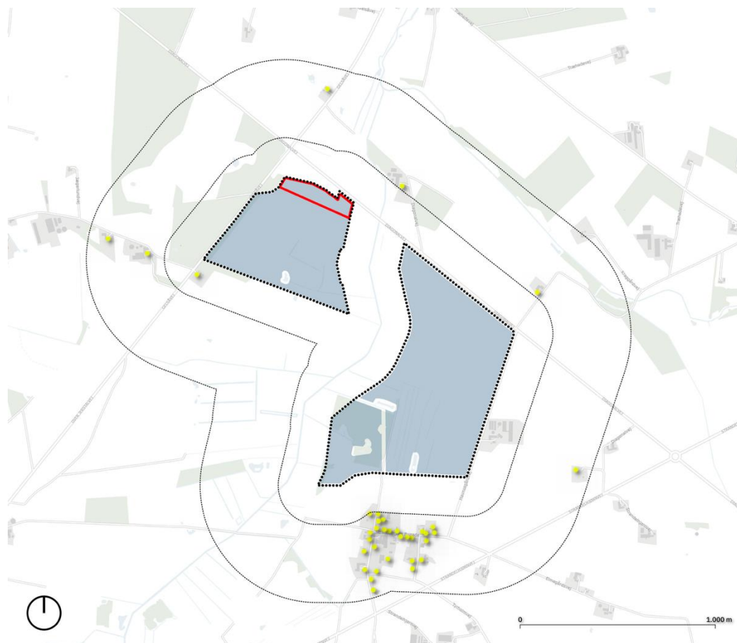
Figur 10.2: Nærmeste naboer til solcelleprojektet er markeret med gul farve. Områder hvor der kan opføres solcelleanlæg er vist med blå flade. Byggefelter hvor der kan opføres batterianlæg, step-up transformer og solceller er vist med rød streg. Sorte stiplede linjer viser en afstand på hhv. 200 meter og 600 meter fra solcelleprojektets områdefafgrænsning. Solcelleprojektets områdefafgrænsning er vist med sort prikket linje.
