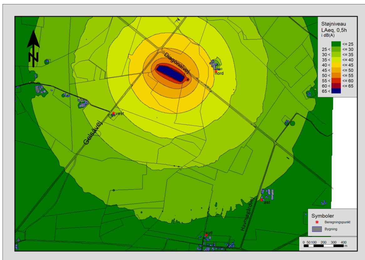
Figur 3b. Støjkonturkort 1,5 m. over terræn i natperioden med beregningspunkter.
