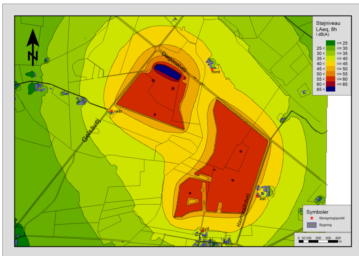
Figur 3a. Støjkonturkort 1,5 m. over terræn i dag/aftenperioden med beregningspunkter.
