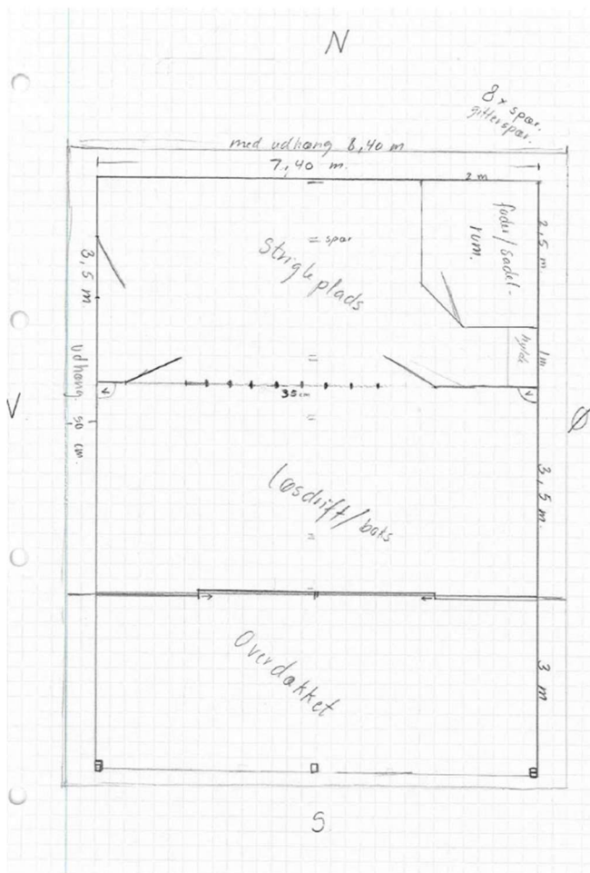
Plantegning af stald
