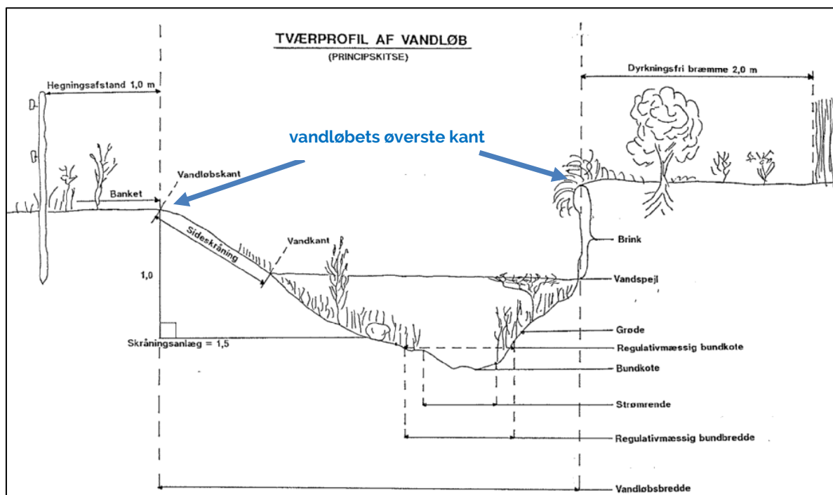
Figur 1. Skitse af tværprofil af vandløb, der bl.a. viser hvorfra man måler afstanden fra vandløbets øverste kant. Skitsen stammer fra vandløbsregulativet for Ulvkærbæk.
