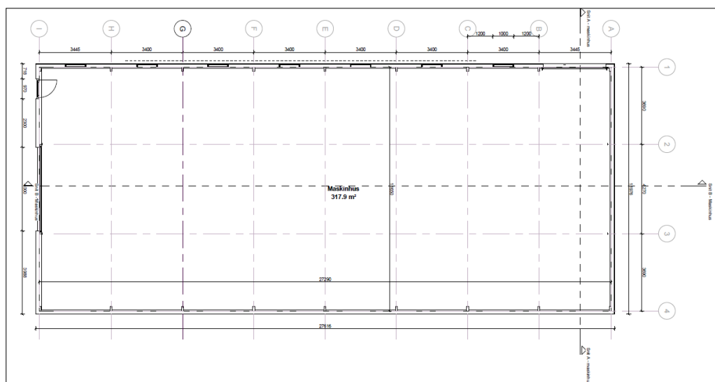
Fra ansøgningen: Plantegningen
