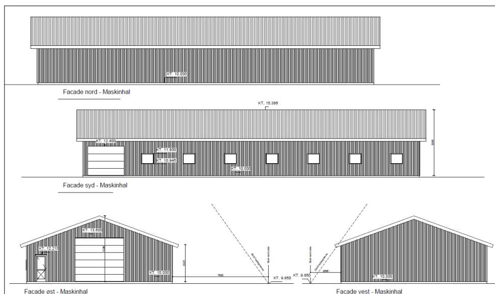
Fra ansøgningen: Facadetegninger af hallen
