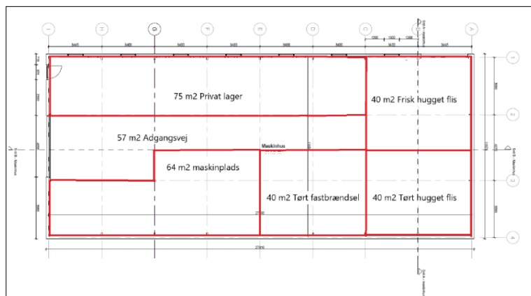
Fra ansøgningen: Plantegningen
