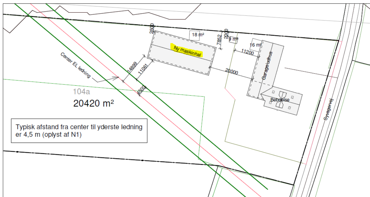
Fra ansøgningen: Situationsplan – Den lyserøde linje viser midten af højspændingsledningerne/masterne på ejendommen
