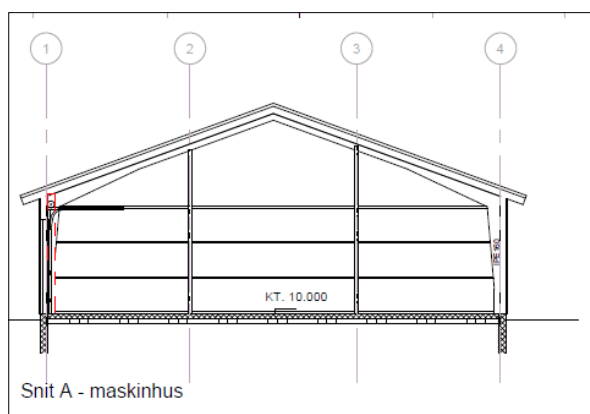
Fra ansøgningen: Tværnsnit af hallen
