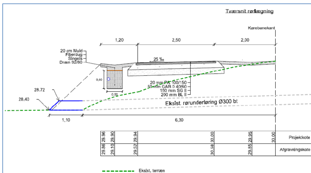
Figur 2. Figuren viser den nye cykelsti samt de nuværende terrænforhold med grønt og det forlængede rør med blåt.
