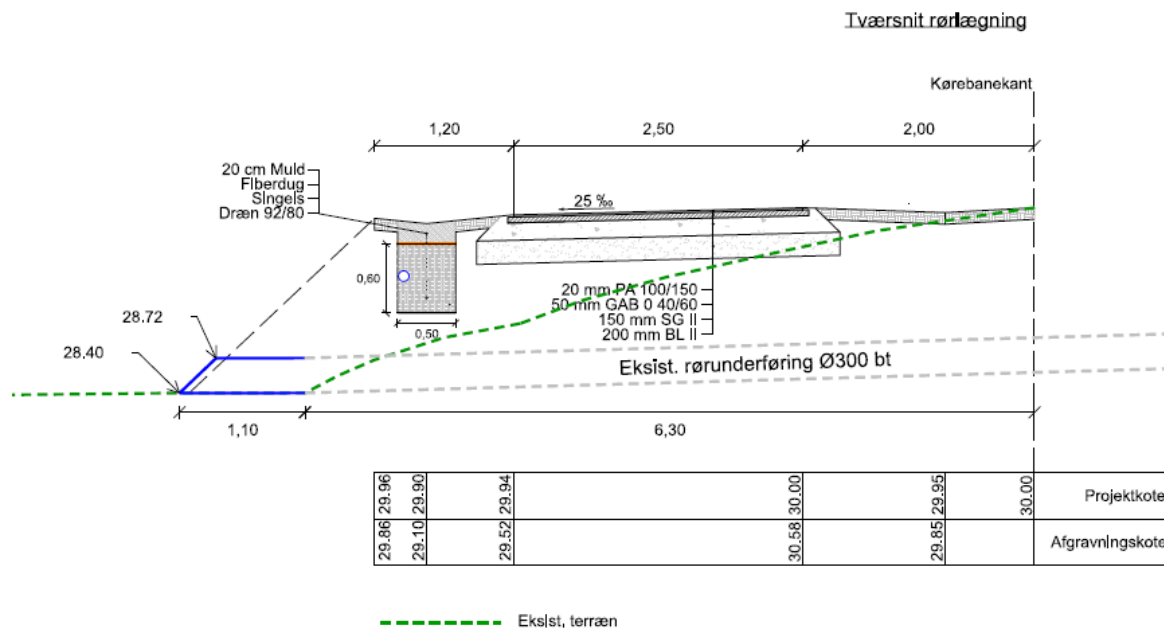
Figur 3: Rørunderføringens placering under den kommende cykelsti
